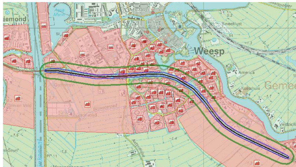
Figuur 4.1 Ligging plaatsgebonden risicocontouren: blauw = 10 -7 , groen = 10 -8
